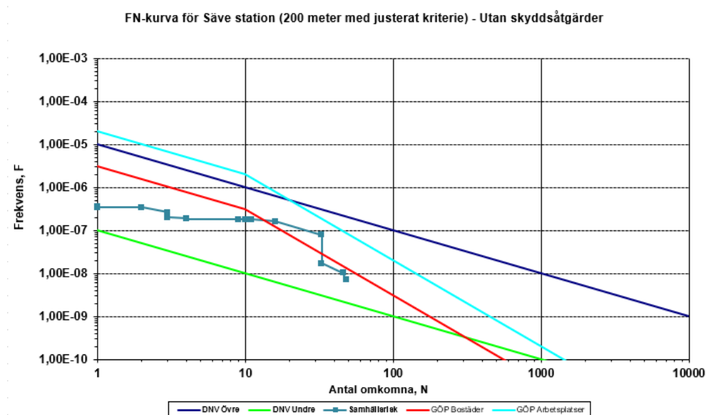
Figur D.1. Samhällsrisk för studerat område (ny och befintlig bebyggelse). Samhällsrisk baseras på uppgifter från Trafikverket samt att mängden farligt gods på Bohusbanan antas öka med 20% från 2017 till 2040.
