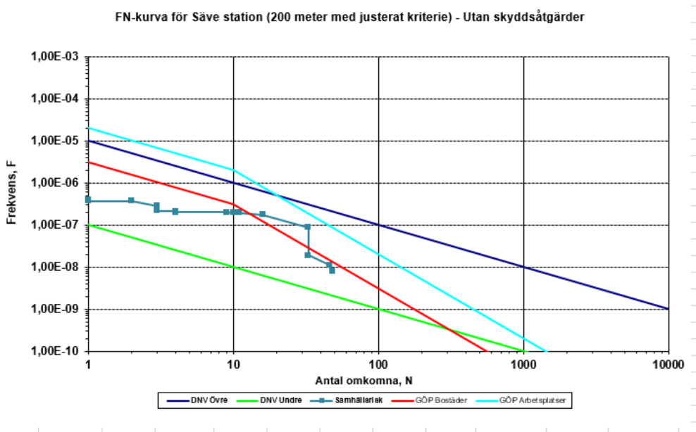
Figur 11. Samhällsrisken för studerat planområde efter etablering i enlighet med beskrivningar i kapitel 3, utan hänsyn till riskreducerande åtgärder.
